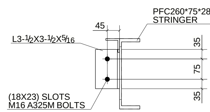
SECTION - 1P - 1P
