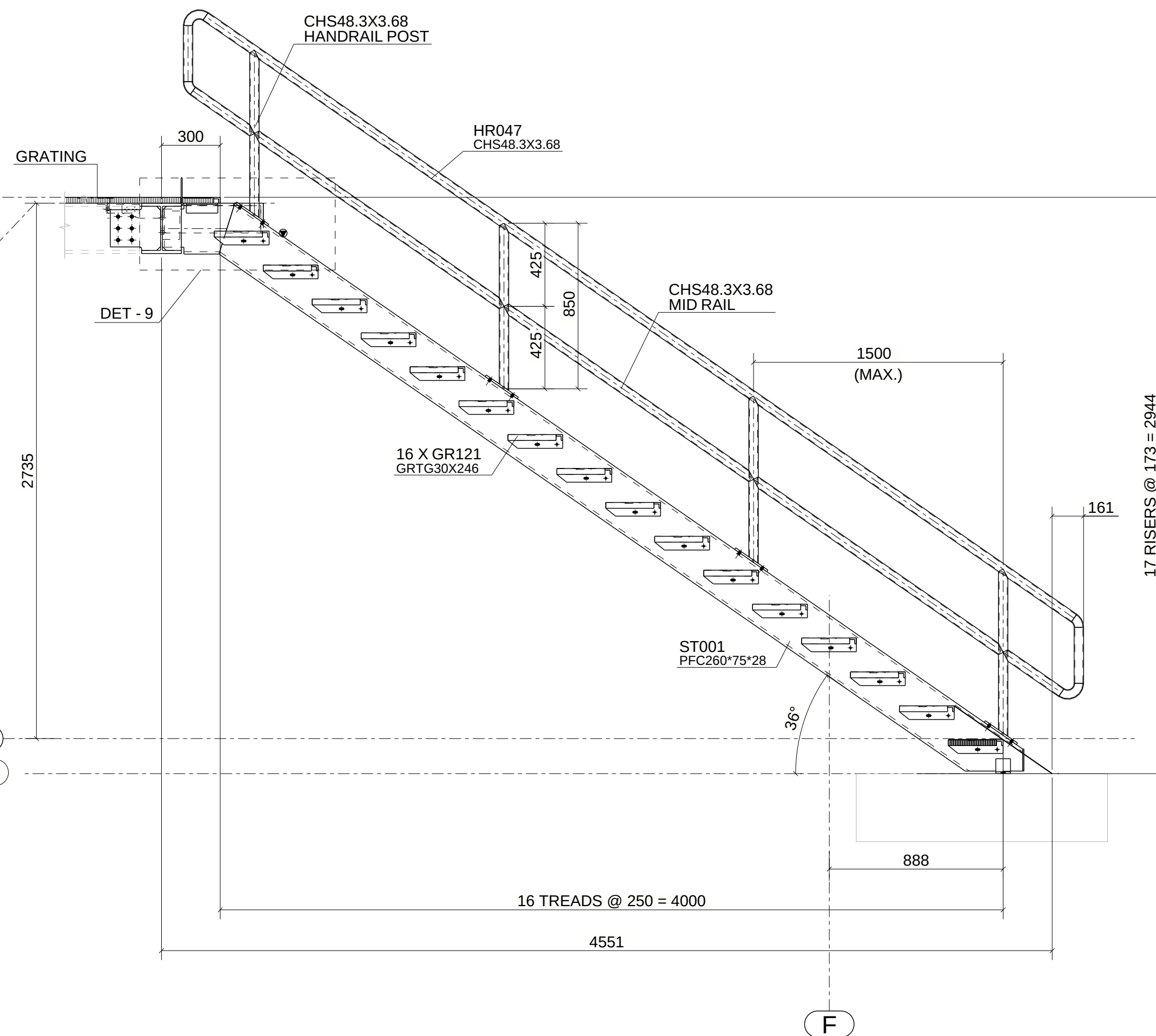
SECTION - AC - AC
